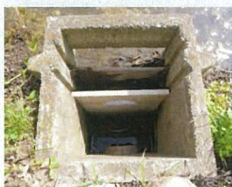
流出を抑制する落水量調整装置の例
